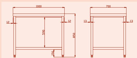
Beispiel: Arbeitstisch mit Grundboden 100x700x850mm
