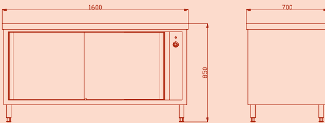
Beispiel: Umluft-Wärmeschrank mit Schiebetüren, 1600x700x850mm
